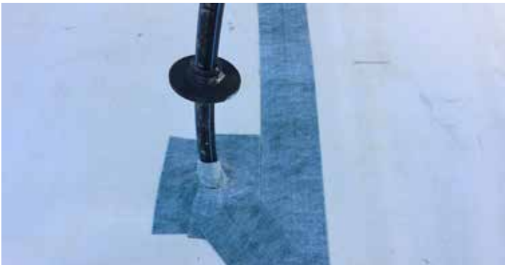
Bild 3: Abdichtung von Durchdringungen mit SikaProof® Tape-150
