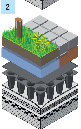
Aufbau Nophadrain Extensives (1) und Intensives (2) Gründachsystem
