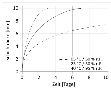
Diagramm 1: Aushärtengeschwindigkeit Sikasil® WS-605 S
