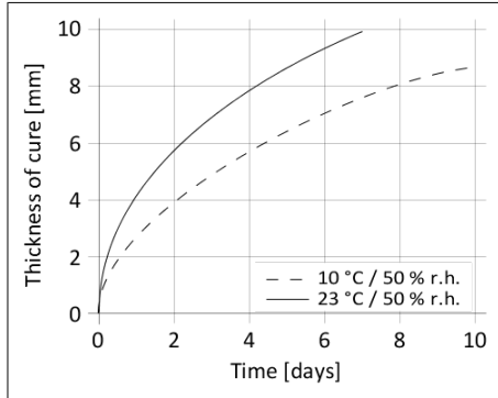
Diagramm 1: Durchhärteschwindigkeit von Sikaflex®-223
