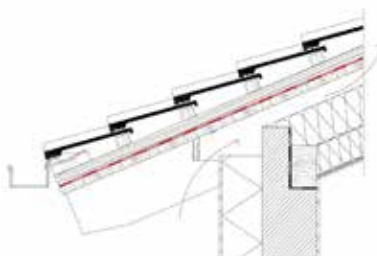
Detail Zwischen-sparrendämmung | Unterdach im Traufenbereich
