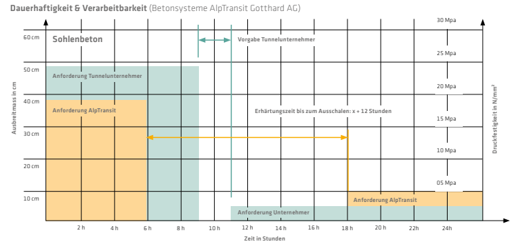
Grafik: Betonanforderungen bezüglich Verarbeitungszeit und Frühfestigkeitsentwicklung (Vorgabe AlpTransit und die Anforderungen des Tunnelbauunternehmers)
