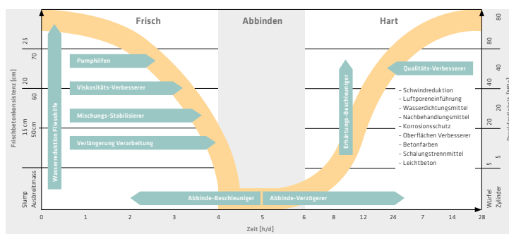
Grafik: Übersicht der Betonzusatzmittelanwendungen zur Steuerung der Frisch- und Festbetoneigenschaften
