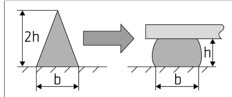
Abbildung 1: Empfohlener Klebstoffauftrag
