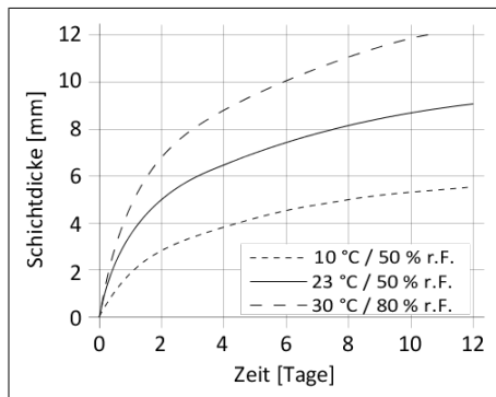
Diagramm 1: Durchhärtgeschwindigkeit von Sikaflex®-260 N
