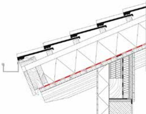
Detail Aufsparrendämmung Unterdach im Traufenbereich
