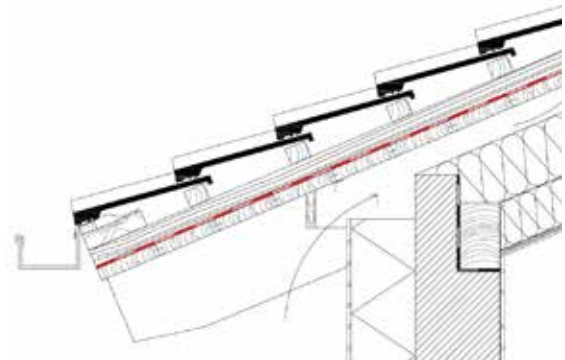
Detail Zwischensparrendämmung Unterdach im Traufenbereich
