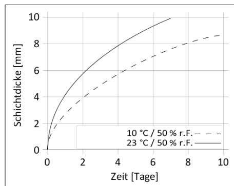
Diagramm 1: Durchhärtegeschwindigkeit SikaTack® MAX 30 (Purform®)
