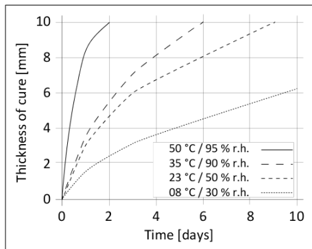
Diagramm 1: Aushärtageschwindigkeit Sikasil® SG-20
