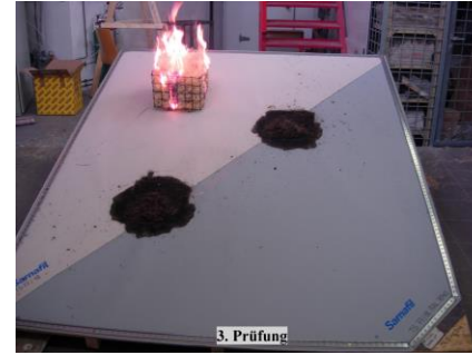
3. Brandversuch
