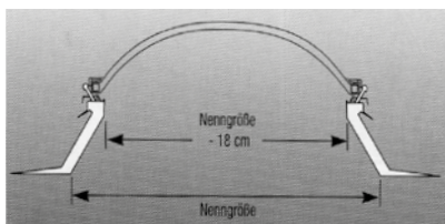
Essexfix® 4000 - starr
