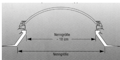
Esstertop® 4000 - belüftbar
